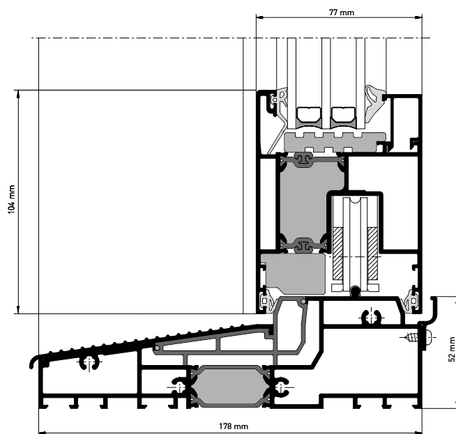
heroal S 77 HI Schnittdarstellung Bodenschwelle zweispurig (HS-Flügelprofil 77/104)
