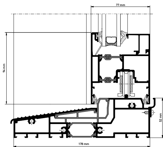
heroal S 77 Schnittdarstellung Bodenschwelle zweispurig (HS-Flügelprofil 77/94)
