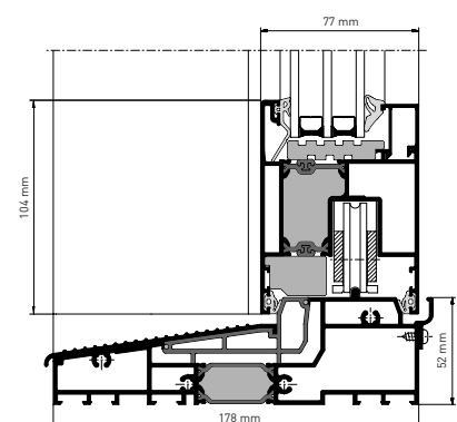
heroal S 77 HI (HS-Flügelprofil 77/104)
