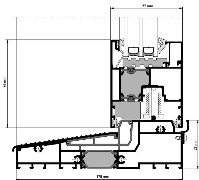
heroal S 77 HI Schnittdarstellung Bodenschwelle zweispurig (HS-Flügelprofil 77/94)
