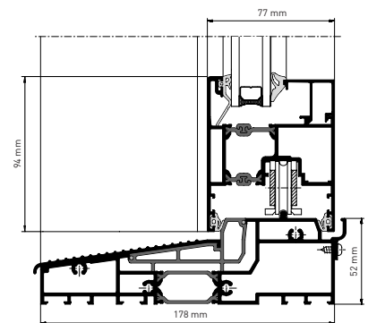
heroal S 77 (HS-Flügelprofil 77/94)
