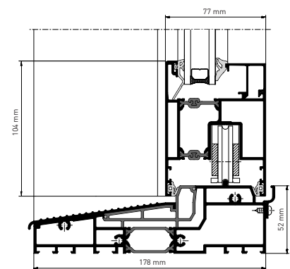
heroal S 77 (HS-Flügelprofil 77/104)
