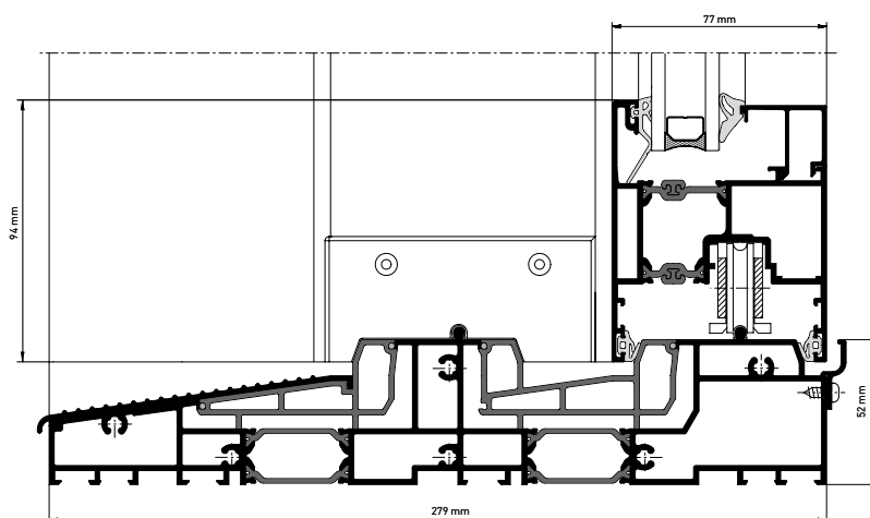
heroal S 77 Schnittdarstellung Bodenschwelle dreispurig (HS-Flügelprofil 77/94)
