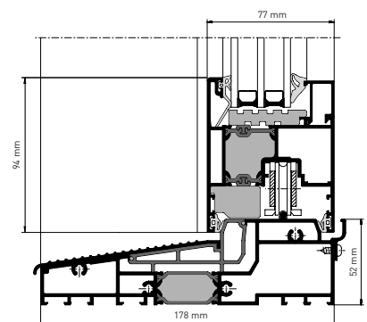
heroal S 77 HI (HS-Flügelprofil 77/94)
